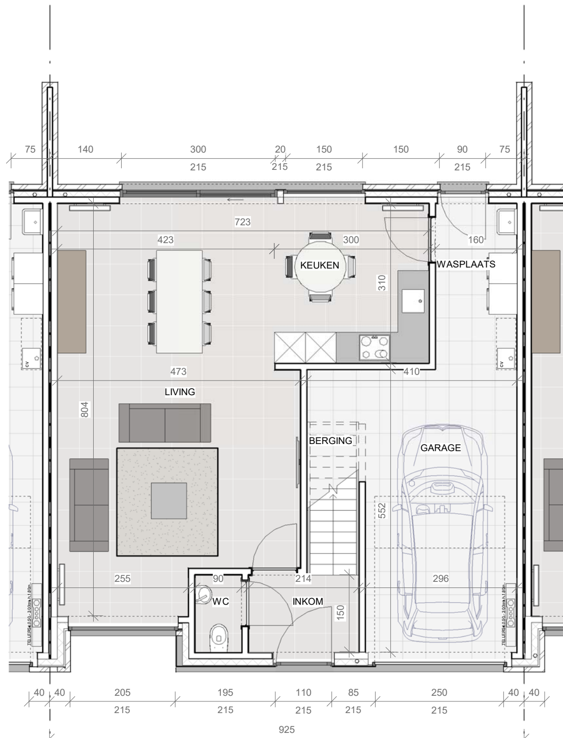
LOT 10 GELIJKVLOERS
