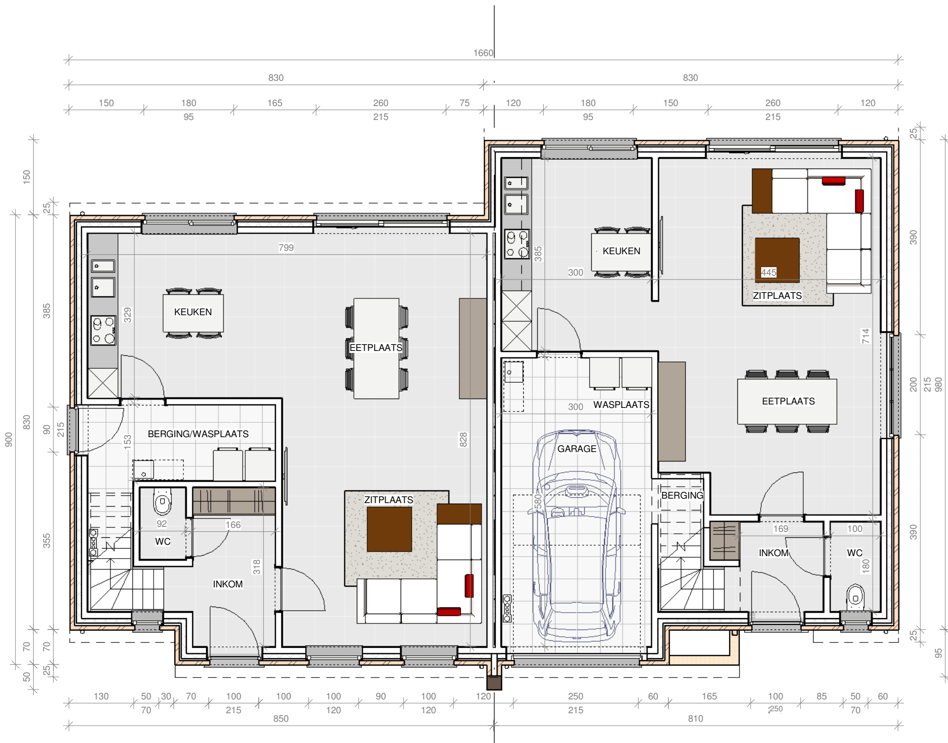
GELIJKVLOERS LOT 14
