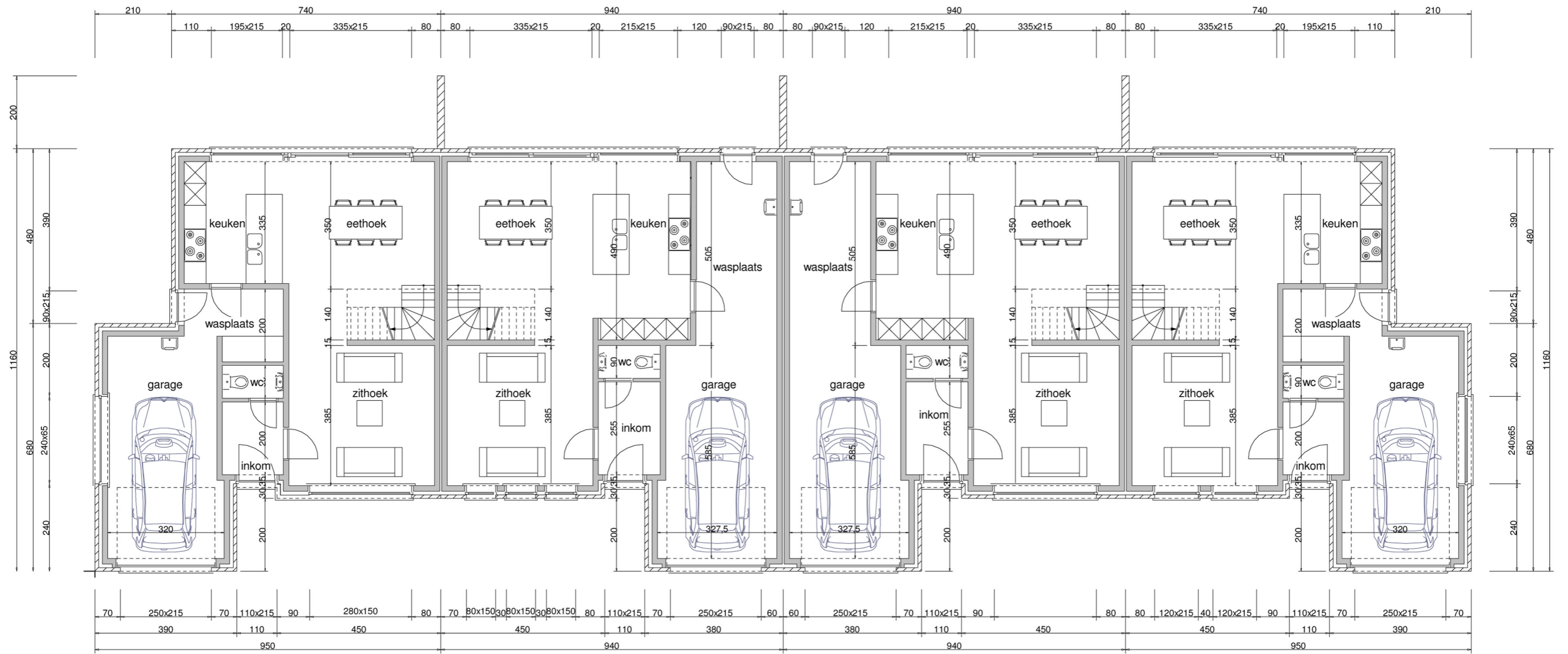
GELIJKVLOERS LOT 1
