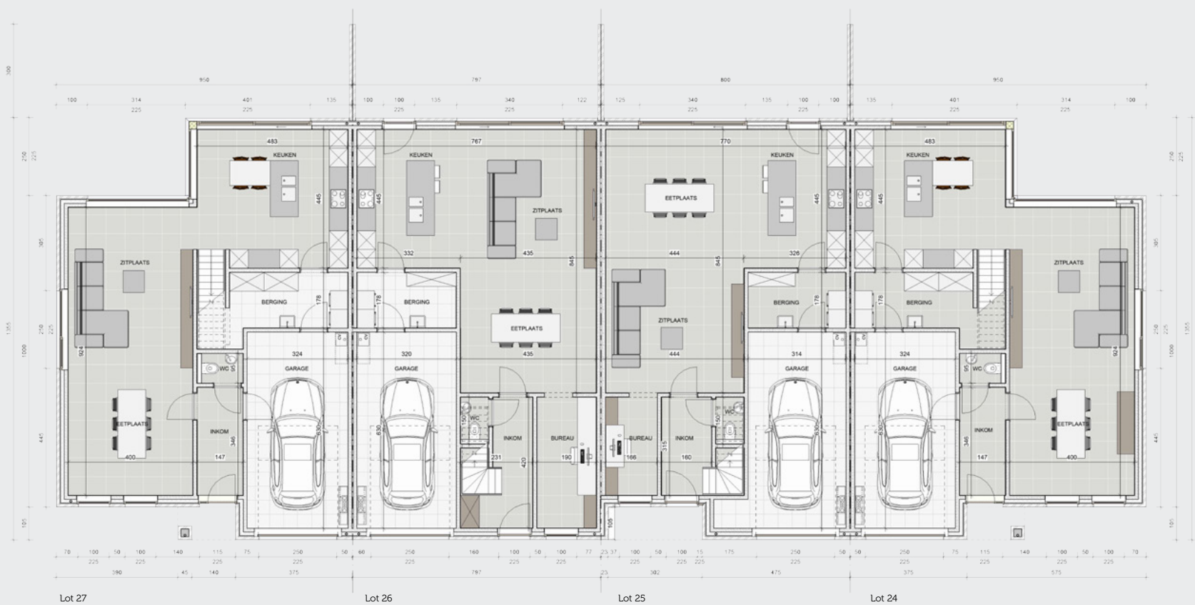
Gelijkvloers
