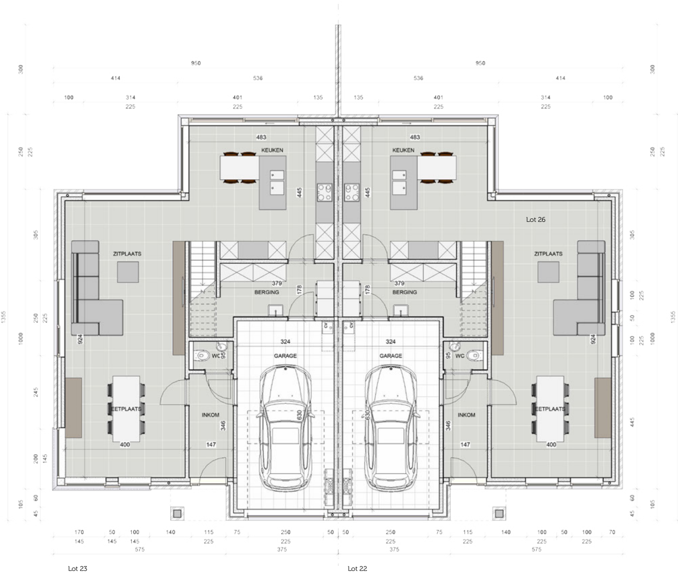
Gelijkvloers
